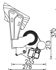
Montaggio sottotetto Under-roof installation
