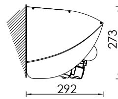
Montaggio sottotetto Under-roof installation
