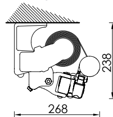
Montaggio a soffitto Ceiling installation
